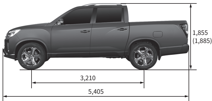
측면
